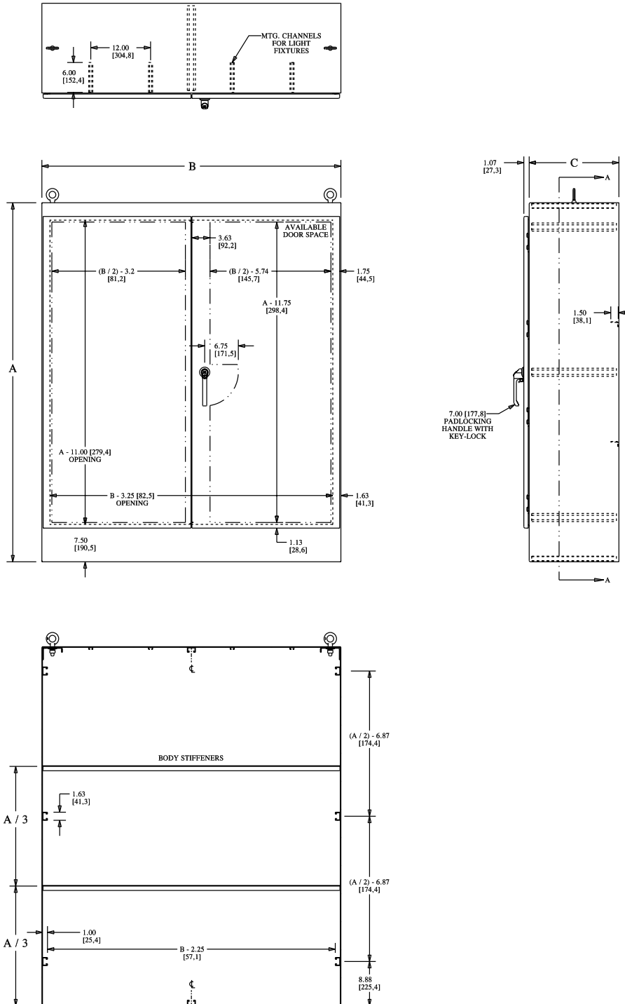
SECTION A-A
